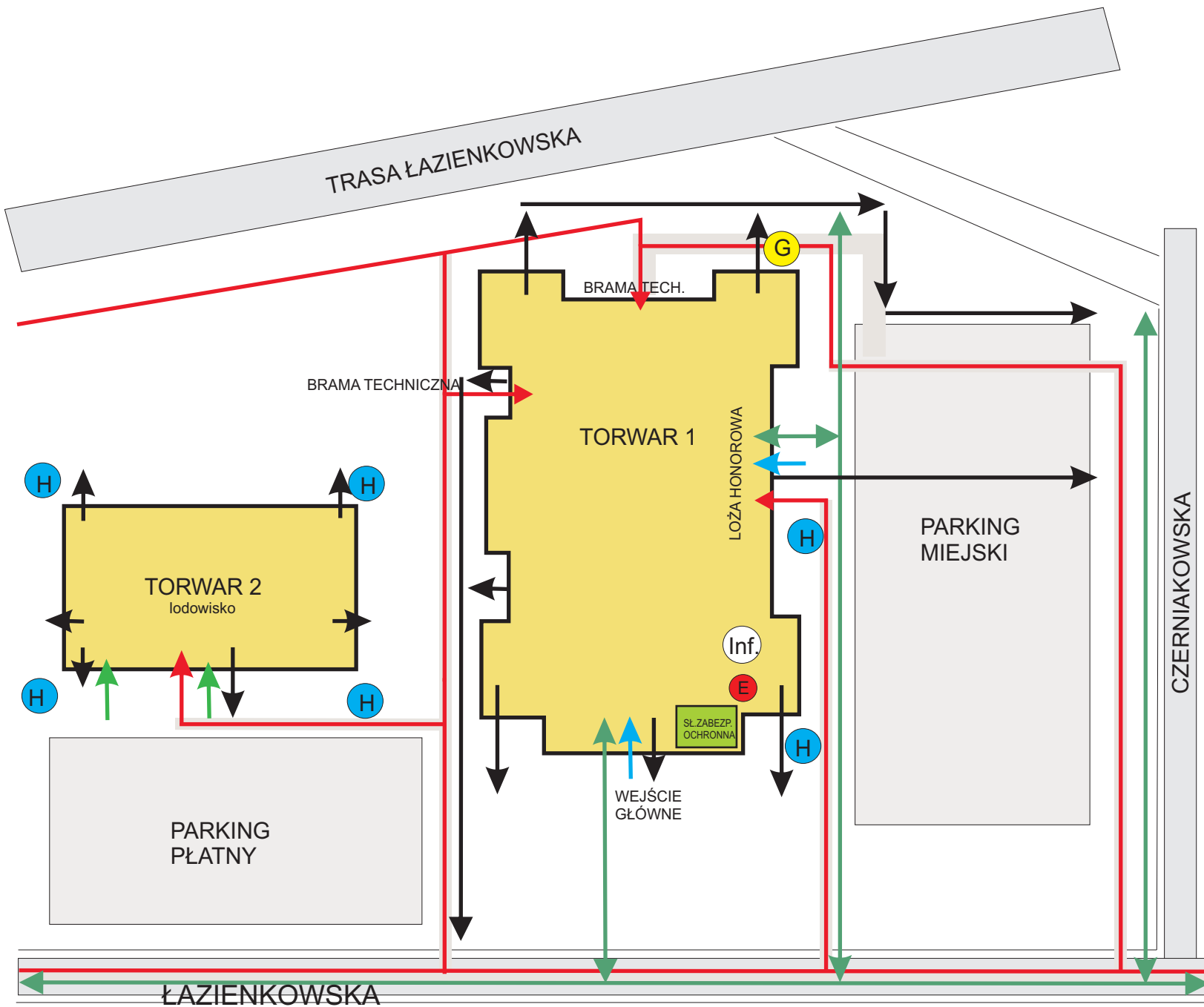
PLAN SYTUACYJNY OBIEKTÓW TORWAR - DROGI DOJAZDOWE I EWAKUACYJNE DLA SŁUŻB RATOWNICZYCH
